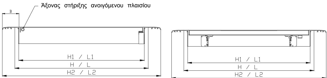
ACDR - ΤΟΜΕΣ
