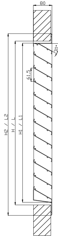
FA-450 – ΤΟΜΗ
