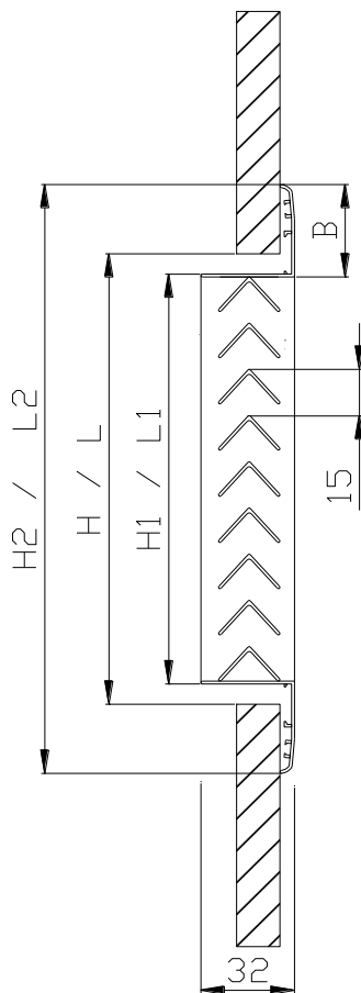
RD-301 - SECTION
