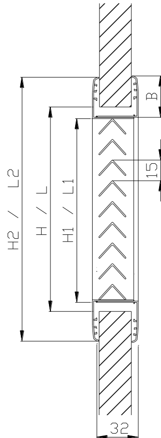
RD-302 - SECTION
