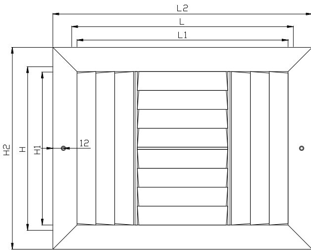
CM-504 – ΟΨΗ (L x H)
