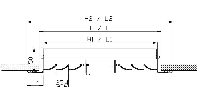
CM-504-E – TOMH ME ΕΣΧΑΡΑ
