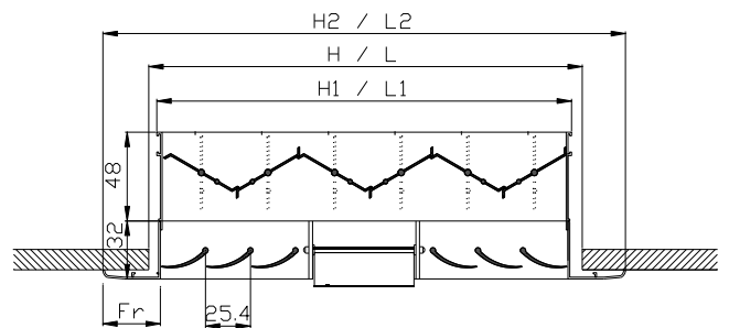
CM-504-D – TOMH ME DAMPER
