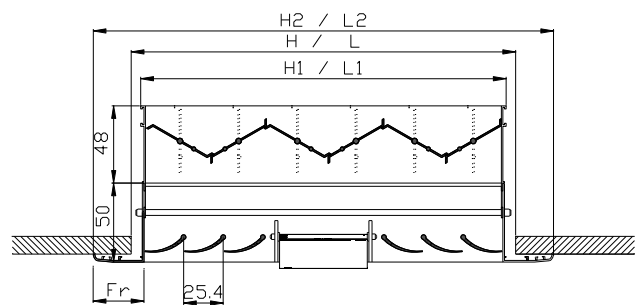
CM-504-D-E – TOMH ME DAMPER ΚΑΙ ΕΣΧΑΡΑ
