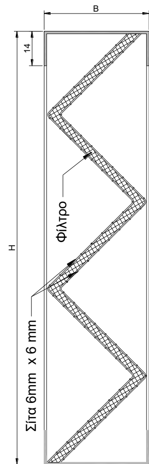
FZ - ΤΟΜΗ
