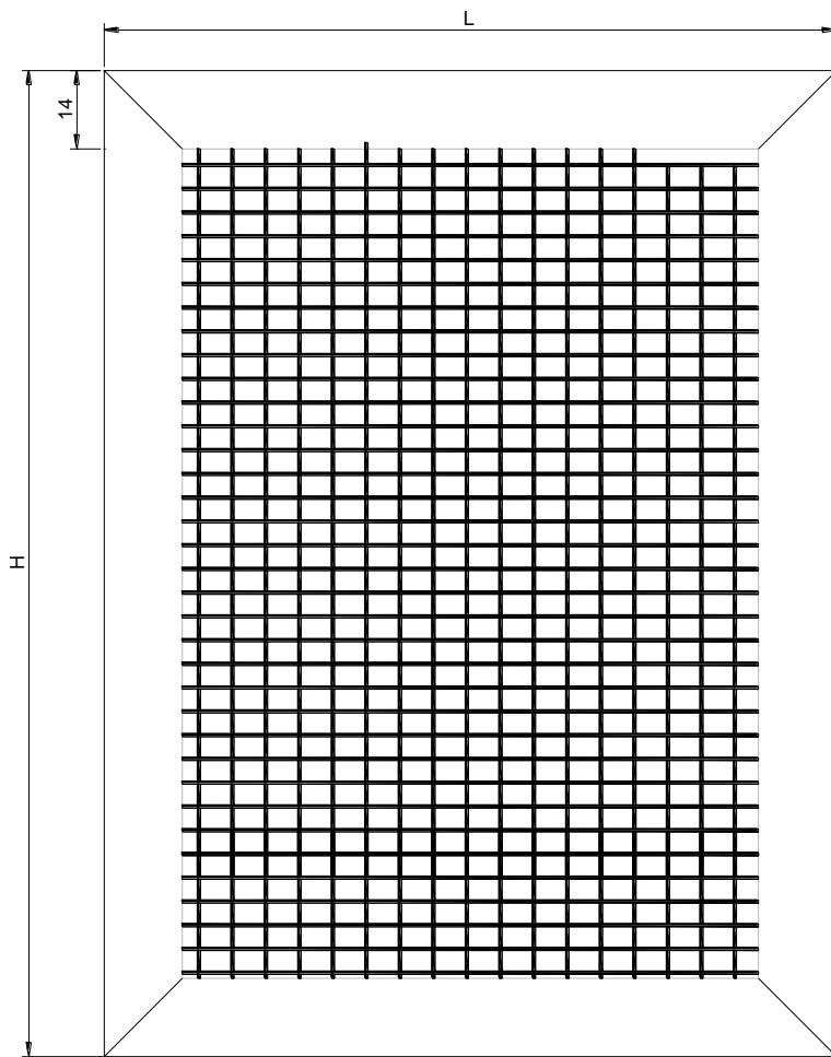
FZ - ΟΨΗ
