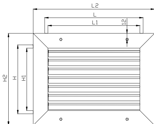
WR-150 – ΟΨΗ (L x H)
