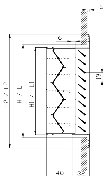
WR-150-D – TOMH ME DAMPER
